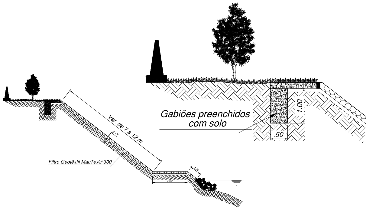
Seção Transversal Típica
