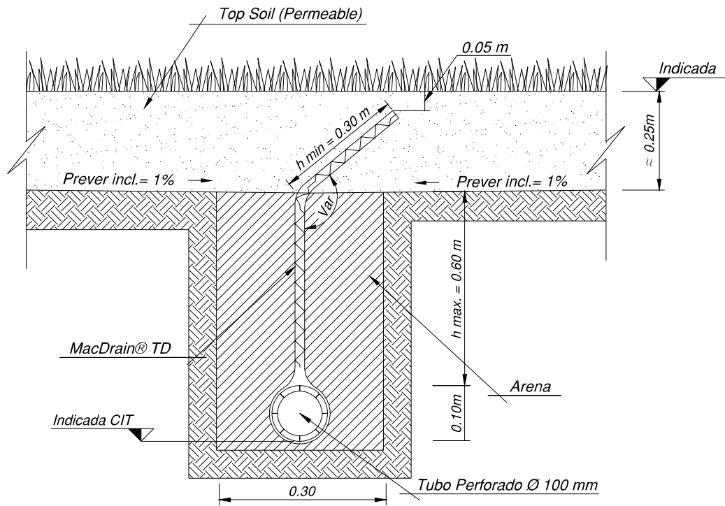
Sección Transversal Típica
